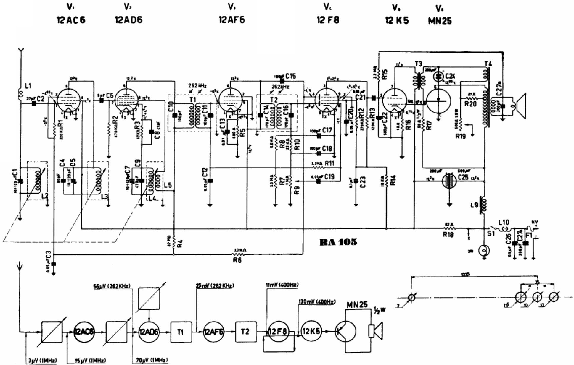
AUTOVOX - Mod. RA '105. Apparecchio con valvole a tensione anodica di 12 volt, e perciò funzionante senza vibratore e valvola raddrizzatrice. Gamma onde medie da 520 a 1600 kc/s. Stadio finale con un transistor; è sistemato esternamente, sul lato destro, fissato ad una piastra di raffreddamento. Media frequenza a 455 kc/s. Potenza d'uscita 3 watt con dieci per cento di distorsione. Consumo da 2 a 2,4 ampère. (Per Note di Servizio v. quelle dei modd. 101/103).
